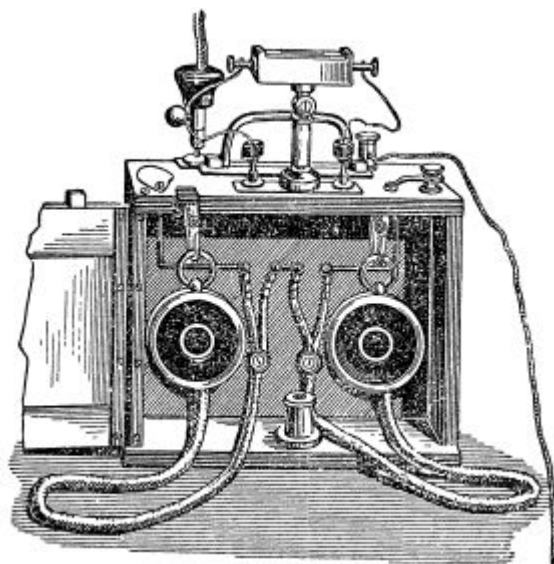
Конструкция приёмника с детектором и телефонными трубками.
