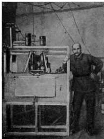
Генератор коротких волн Нижегородской радиолaborатории. Справа — В. В. Татаринов.
