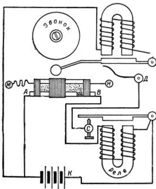
Схема первого радиоприёмника.
