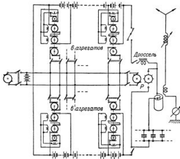
Схема искрового передатчика Ходынской радиостанции.
