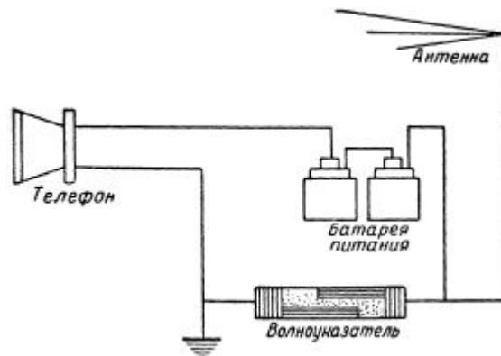
Схема приёмника с телефонной трубкой.
