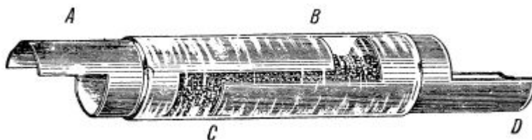
Волнообнаружитель конструкции А. С. Попова.
