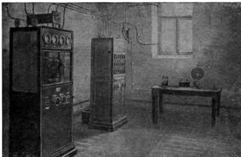
Радиовещательная станция типа «Малый Коминтерн» мощностью 1,2 киловатта.
