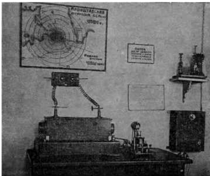
Корабельный радиопередатчик конструкции А. С. Попова.
