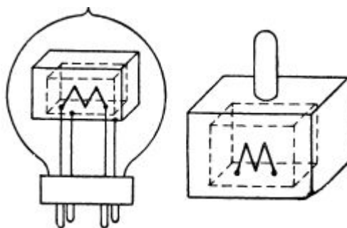
Лампы конструкции В. И. Коваленкова.
