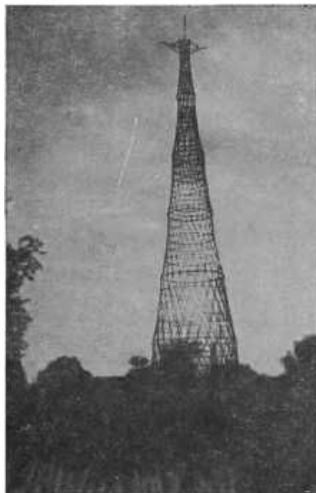
Шуховская башня. Наверху видны антенны телевизионного передатчика и передатчика звукового сопровождения.
